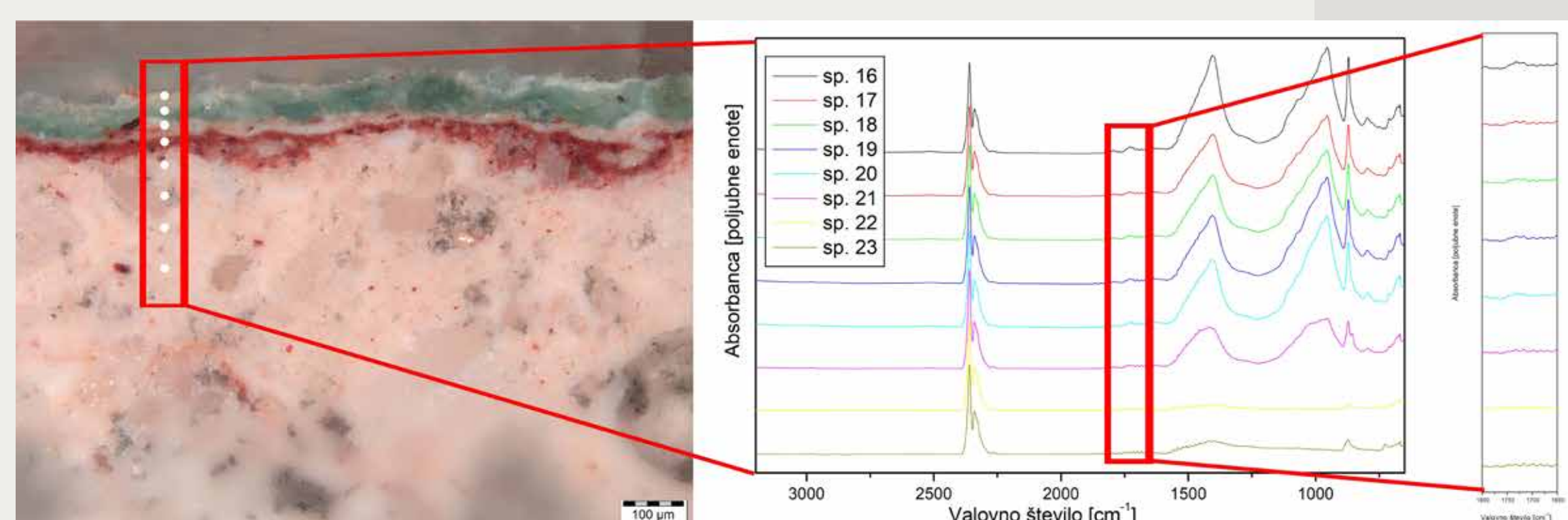
Slika 4: Stratigrafija vzorca, odvzete z ornamenta na sliki 2, in FTIR spektri označenih točk. Na desni je povečano območje karbonilnih vibracij, ki potrjujejo prisotnost voska. (foto: K. Kavkler)
