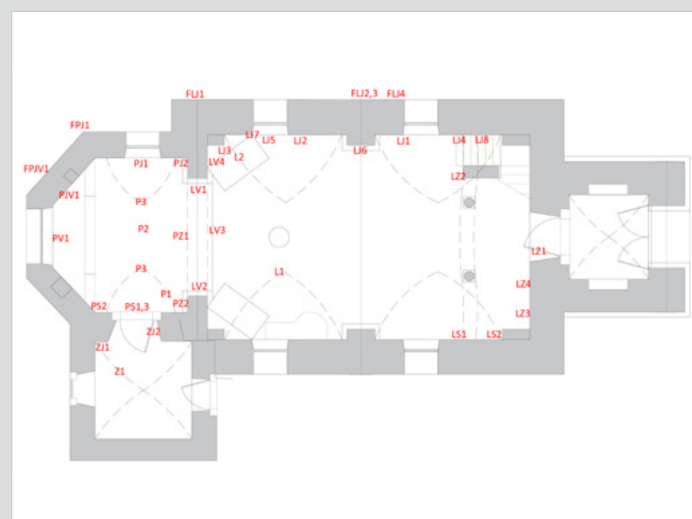
Slika 1: Tloris cerkve s pozicijami sond.
