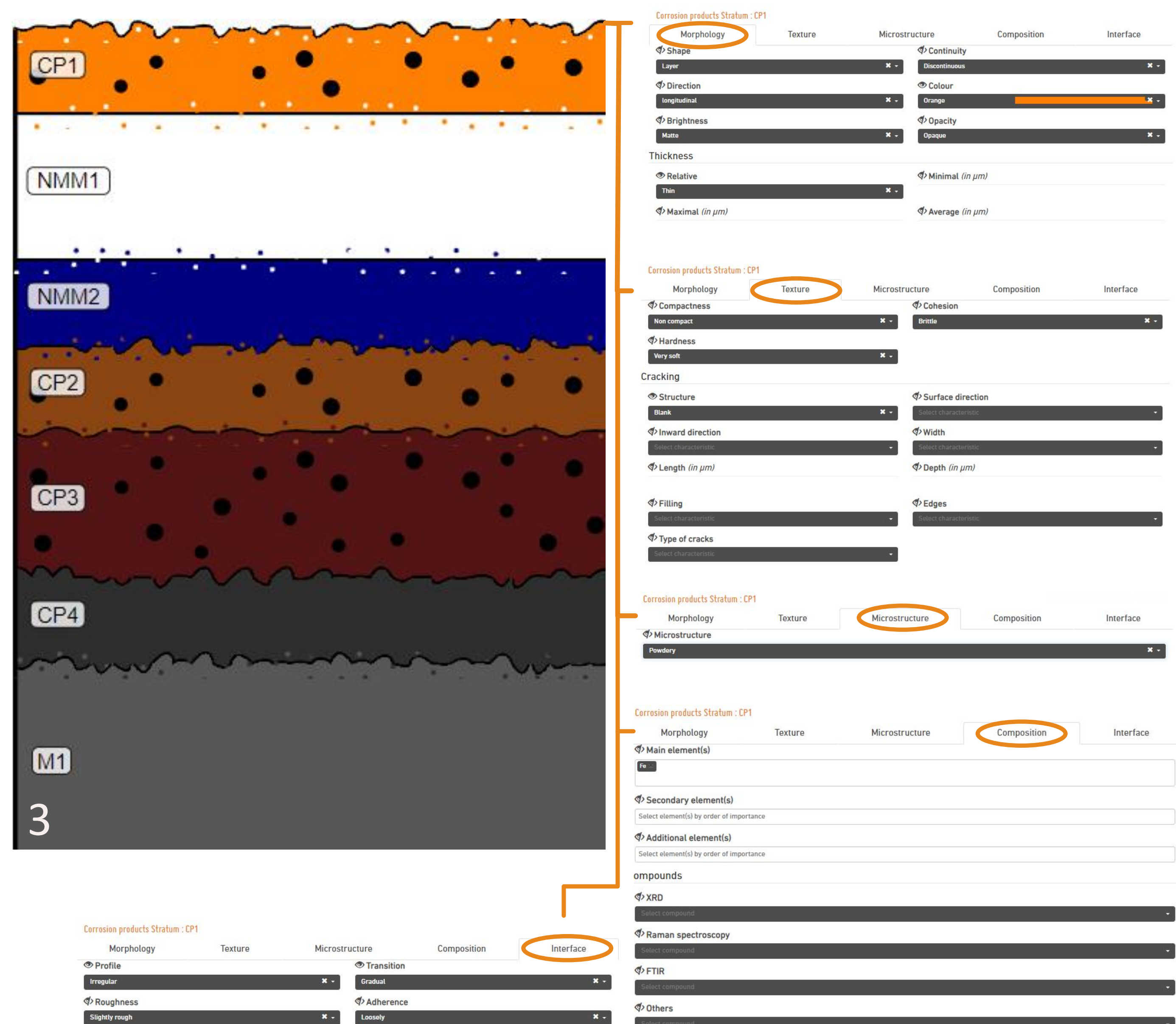
Slika 3: Digitalni prikaz stratigrafije korozijskih produktov na železu (slika 2), izdelan z enim od orodij MiCorr. Vsaka stratifrska plast je opremljena z informacijami o morfologiji, teksturi, mikrostrukturi, kemijski sestavi in značilnostih na stikih posameznih plasti (foto: Zala Uršič)
